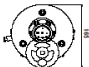
A矢視
