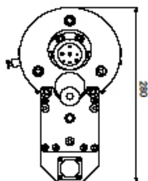
B矢視
