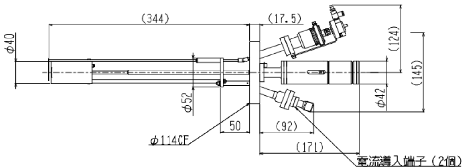
EB蒸着源本体 SSEB-500 (圧空シャッターオプション付き)
