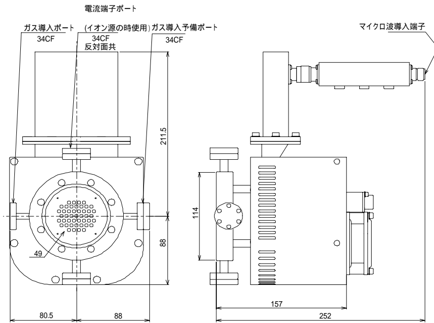
EMIS-221C イオン・ラジカル源本体外観寸法図
