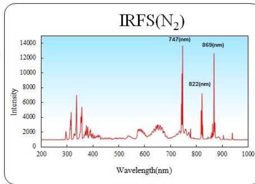
放電スペクトル (窒素) RF電力：300W
