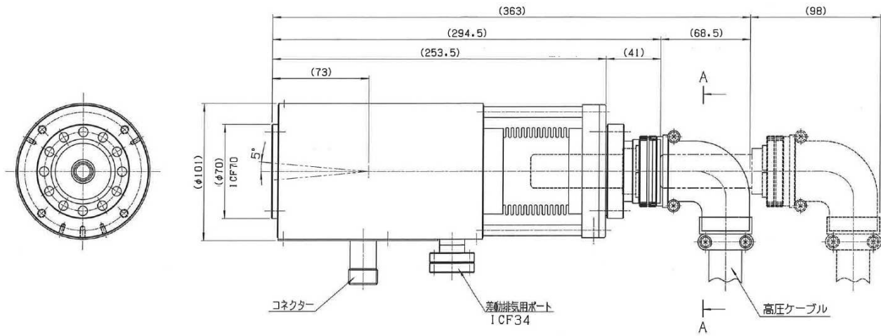
RHEED303-EG 外観寸法図
