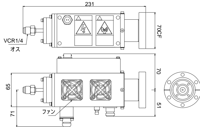
SMPS-201 プラズマ源本体外観寸法図
